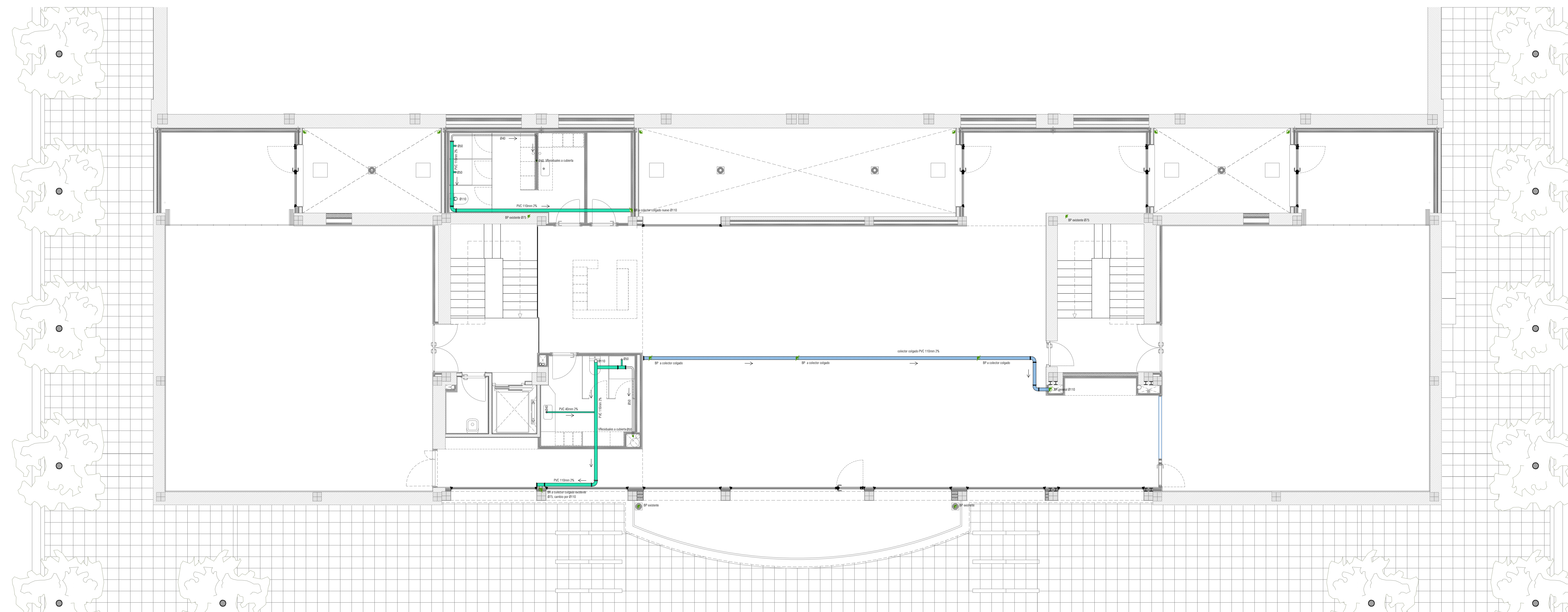
PLANTA PRIMERA
